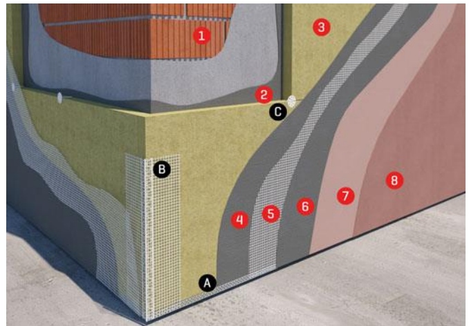
Figura 1. Componentes del sistema Traditerm® mineral
